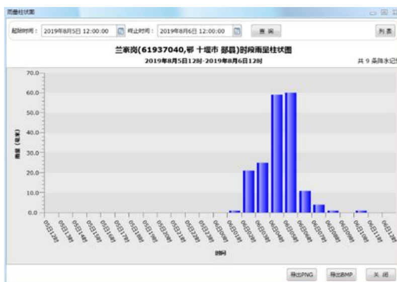
图 3 郧阳区柳坡镇兰家岗站 8.5-8.6 雨量监测图
